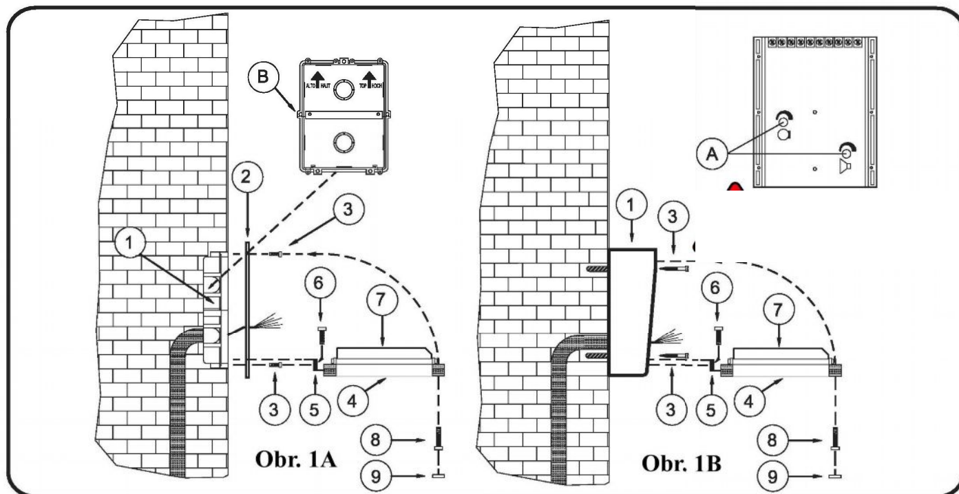
ZAPUŠTĚNÁ MONTÁŽ VENKOVNÍ STANICE (Obr.1A)
