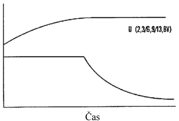
Nabíjecí charakteristika AL 300
