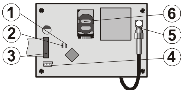
obr. 1 Zapojení komunikátoru
